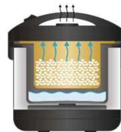
MANTENER CALIDO arroz y almidón ahora separados evaporación final
